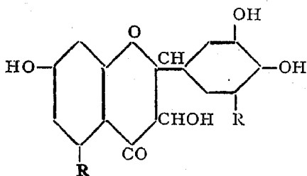
I, R=H
