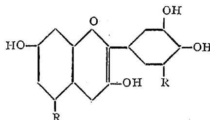
II, R=H
