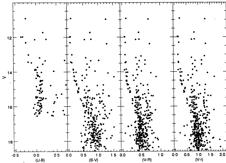
Figure 6. The V , (U - B) ; V , (B - V) ; V , (V - R) and V , (V - I) diagrams for Trumpler 11
