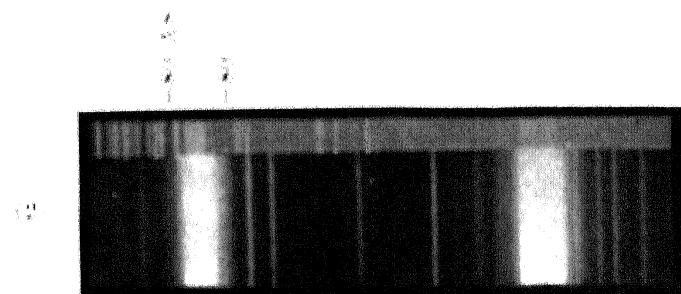
Rhombic Sulphur
