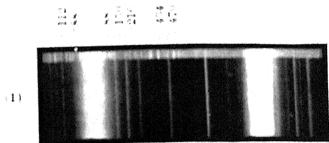
Rhombic Sulphur
