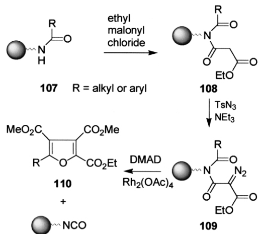
Scheme 31.
