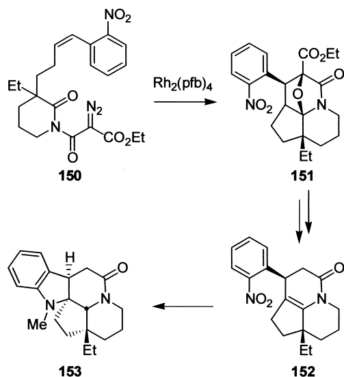
Scheme 45.
