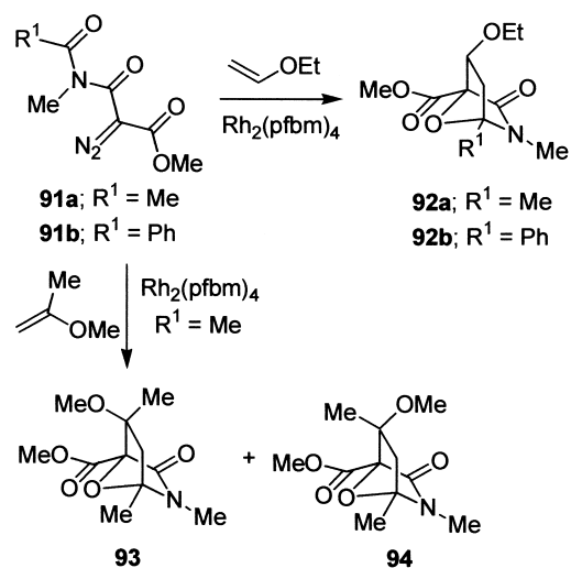
Scheme 27.
