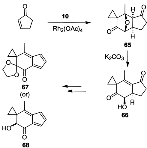
Scheme 20.
