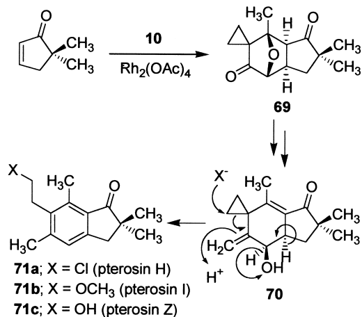
Scheme 21.
