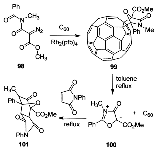
Scheme 29.
