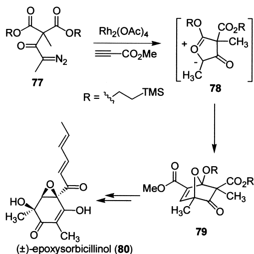
Scheme 23.
